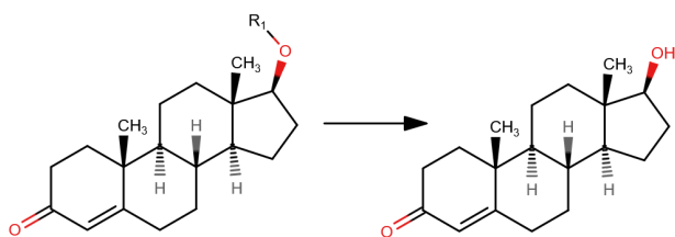
Figure 14 : schéma de la structure des pro-drogues injectables et de leur produit final T
