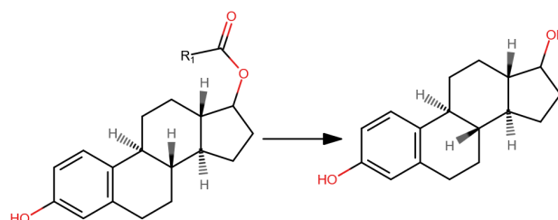
Figure 4 : schéma de la structure des pré-médicaments injectables et de leur produit final E 2 , exception faite du benzoate d'estradiol
